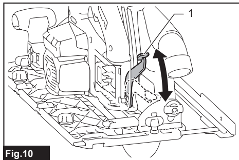
Fig.10 ► 1. Palanca
