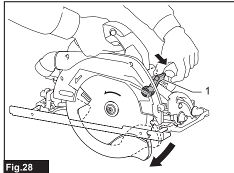
Fig. 28 ► 1. Retracting lever
